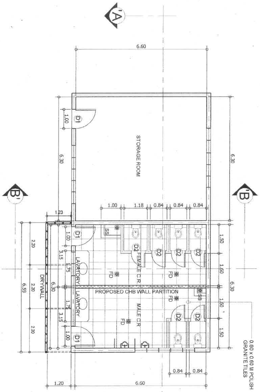
FLOOR PLAN SCALE: 1:100 M
